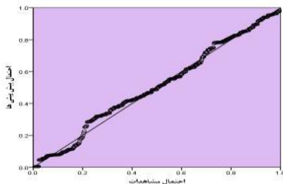
نمودار (۱): نرمال بودن مانده‌ها
