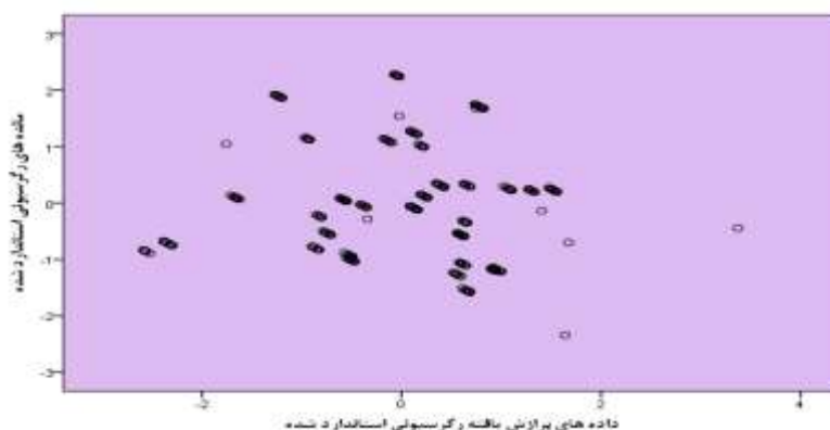
نمودار (۲): ثابت بودن واریانس خطاها
