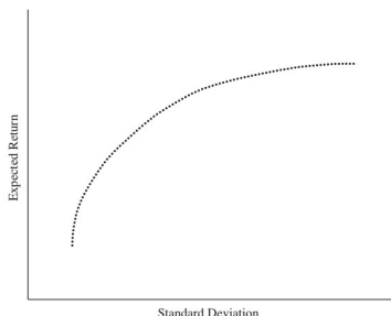
شکل ۱- نمایش نقطه‌ای مرز کارآیی مسئله مارکویتز
