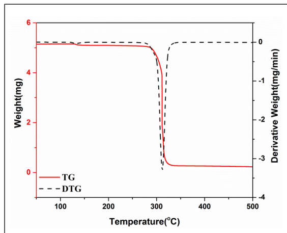
شکل ۷ نمودارهای TG و DTG نانو چندسازه MnC_2O_4 \cdot 2H_2O/AP
