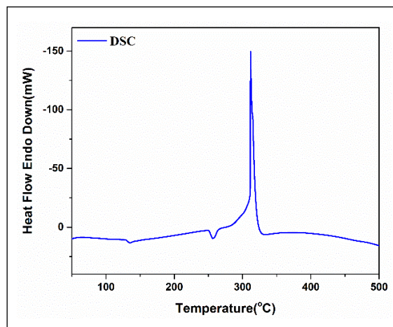
شکل ۸ نمودار DSC نانو چندسازه \text{Mn}_2\text{O}_4 \cdot 2\text{H}_2\text{O}/\text{AP}
