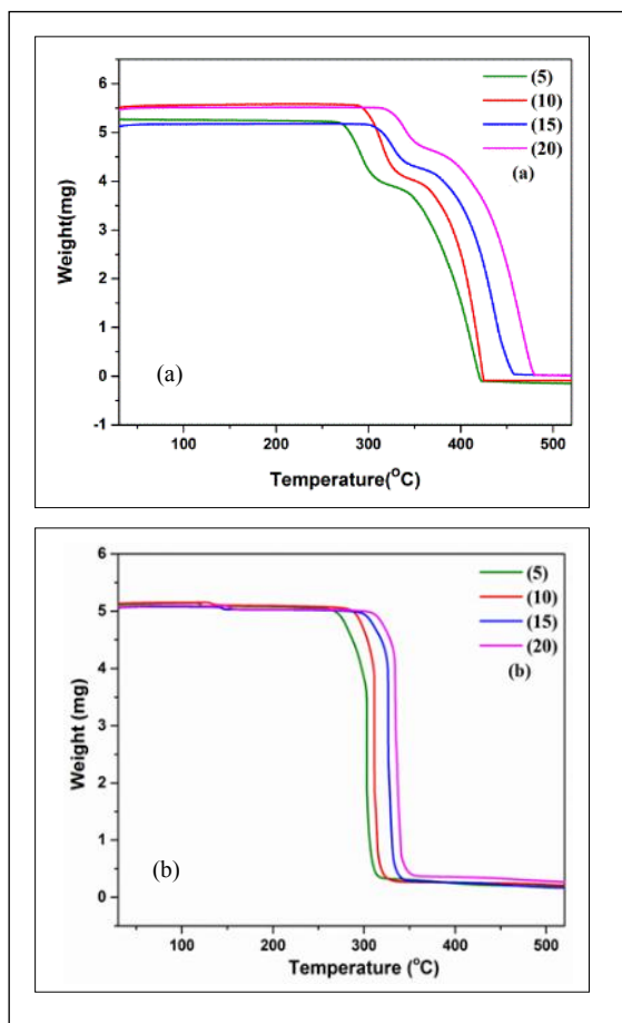
شکل ۹ نمودار TG آمونیم پرکلرات خالص (a) و نانو چندسازه \text{Mn}_2\text{O}_4 \cdot 2\text{H}_2\text{O}/\text{AP} در سرعت‌های متفاوت گرمادهی ۵، ۱۰، ۱۵ و 20^{\circ}\text{C}/\text{min}
