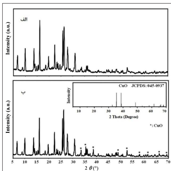
شکل ۲ الگوی پراش پرتو ایکس زئولیت (الف) موردنیت تهیه‌شده و (ب) نانوچندسازه موردنیت-CuO
