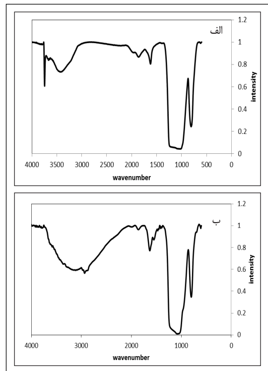
شکل ۱۱ (الف) طیف فروسرخ نمونه SBA-15 و (ب) طیف فروسرخ نمونه SBA-15-NH₂
