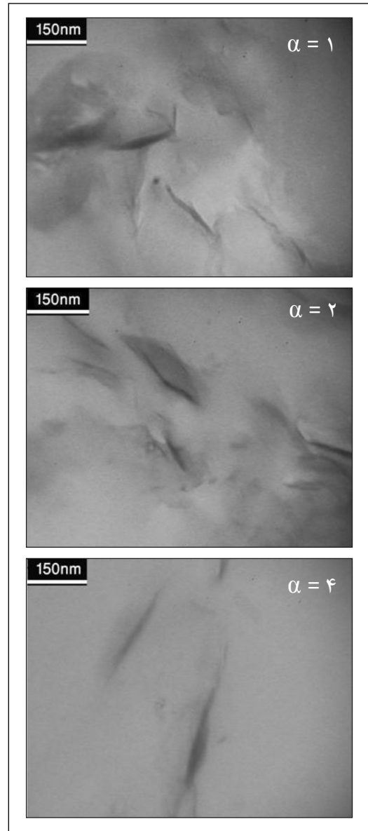
شکل ۷ تصویرهای میکروسکوپ الکترونی عبوری نانوکامپوزیت‌های تولید شده با نسبت‌های کشش ۱، ۲ و ۴
