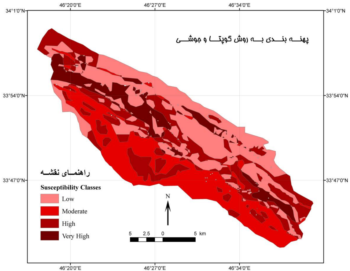
تصویر ۶- نقشه پهنه‌بندی خطر زمین لغزش به روش گوپتا و جوشی
