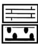
تصویر ۲- ستون چینه‌نگاری سنگی برش مورد مطالعه
