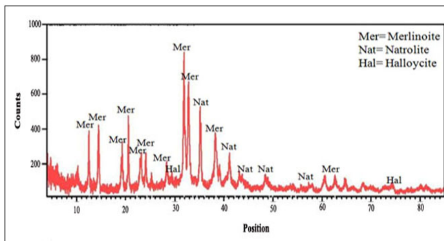
تصویر ۴- پیک‌های Mer: مرلینوئیت، Nat: ناترولیت و Hal: هالویسیت بر روی الگوی XRD
