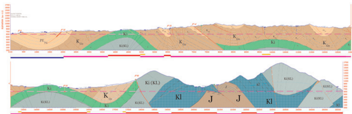
تصویر ۱- مقطع زمین شناسی مسیر تونل (افتخاری و همکاران ۱۳۹۱)
