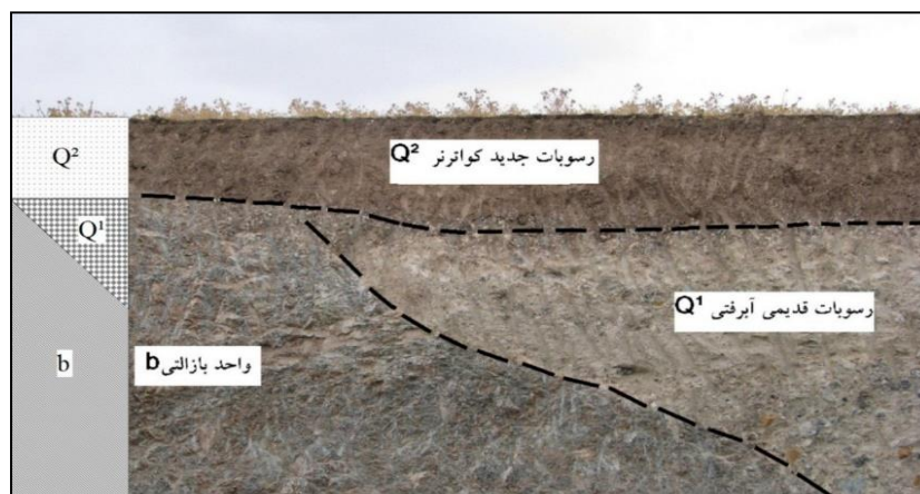
شکل ۳. نحوه ارتباط واحدهای مختلف زمین‌شناسی در محدوده کامیاران (جاده کمربندی، ۱۵۰ متر بالاتر از ترمینال اصلی شهر)
