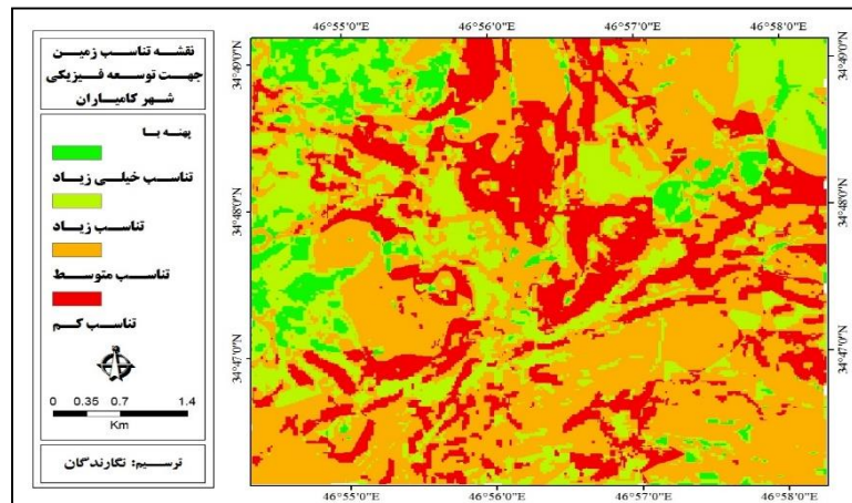
شکل ۱۴. تناسب زمین جهت توسعه فیزیکی شهر کامیاران به روش AHP
