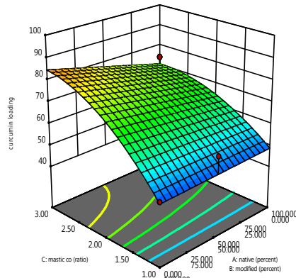
شکل ۲- نمودار سطحی سه بعدی تاثیر صمغ مصطکی اصلاح نشده (A)، اثر صمغ مصطکی اصلاح شده (B) و نسبت صمغ مصطکی به کورکومین (C) بر میزان کارآیی ریزپوشینه کردن در ریزپوشینه‌های صمغ مصطکی حاوی کورکومین.
