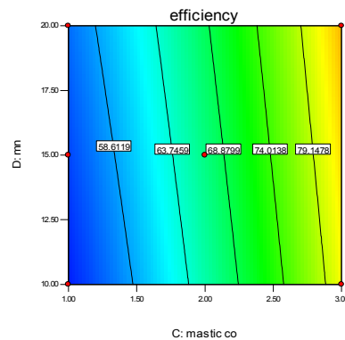
شکل ۳- نمودار سطحی دو بعدی اثر نسبت صمغ مصطکی به کورکومین (C) و میزان منیزیم استنارات (D) بر میزان کارآیی ریزپوشینه کردن در ریزپوشینه‌های صمغ مصطکی حاوی کورکومین.
