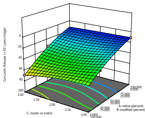
شکل ۹- نمودار سه بعدی اثر صمغ مصطکی اصلاح نشده (A)، اثر صمغ مصطکی اصلاح شده (B) و نسبت صمغ مصطکی به کورکومین (C) بر نرخ رهایش کورکومین در زمان رهایش ۳۰ دقیقه در محیط شبیه‌سازی شده دهانی.
