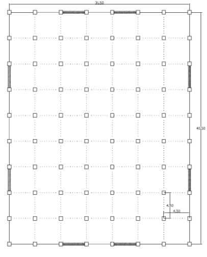
شکل ۵- پلان مدل ۳
