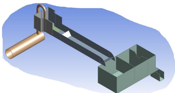
شکل ۲. شماتیک فلوم، ورودی، خروجی و محل نصب دریچه کشوئی
