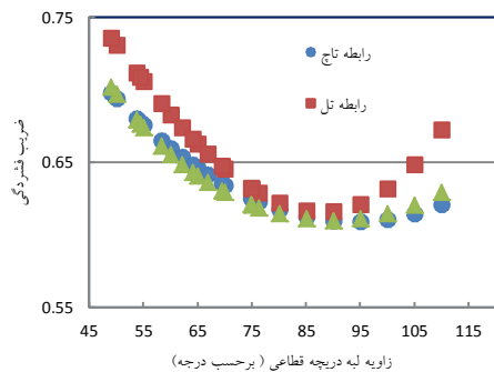
شکل ۷. مقایسه نتایج رابطه نظری پیشنهادی با نتایج روابط محققین پیشین با بکار بردن داده‌های آزمایشگاهی بویالسکی
