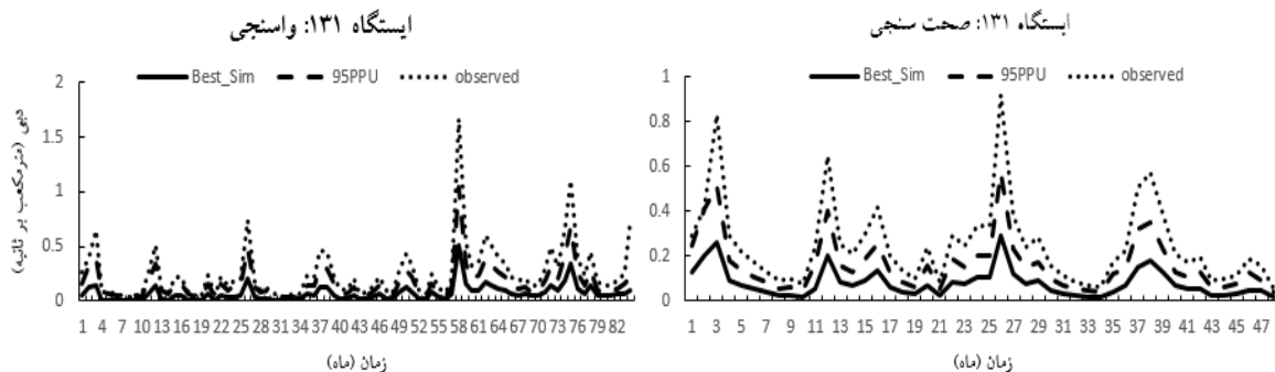
شکل ۶. نتایج واسنجی و صحت‌سنجی ایستگاه شماره ۱۳۱
