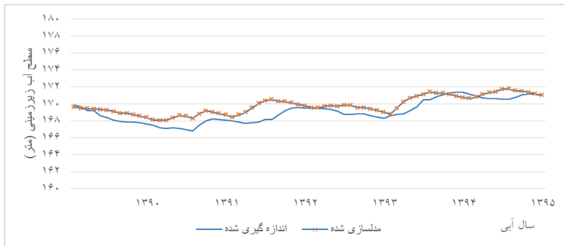
شکل ۴. مقایسه سطح آب زیرزمینی دشت مهران در حالت شبیه‌سازی و اندازه‌گیری شده در مرحله صحت‌سنجی مدل
