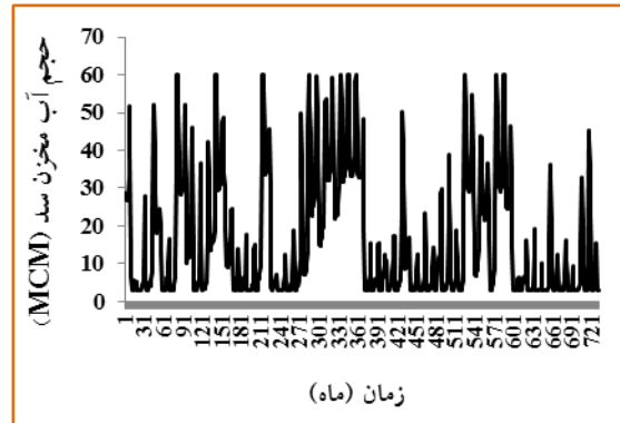
شکل (۹): شبیه سازی تغییرات حجم آب مخزن سد (۱۴۰۰-۱۳۳۹).
