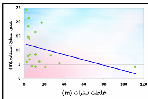
شکل ۳ - رابطه‌ی عمق سطح ایستابی و غلظت نیترات فصل خشک (راست)، فصل تر (چپ).
