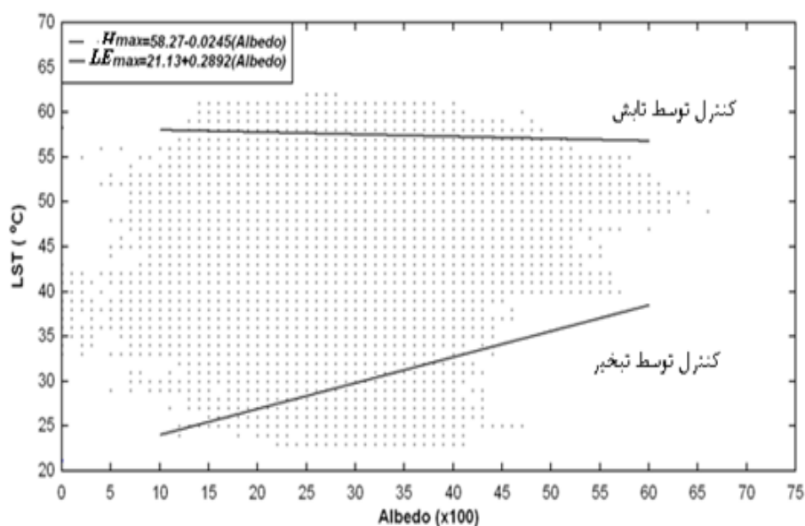
شکل ۲- نمودار پراکنش نقطه‌ای بازتابش- دمای سطح زمین به دست آمده از داده‌های ماهواره‌ای مادیس بر فراز استان اصفهان در یک روز آفتابی (روز گاهشمار قیصری ۲۰۹ سال ۲۰۰۱، برابر با ۳ اوت). محور افقی مقادیر بازتابش سطحی و محور عمودی دمای سطح زمین بر حسب درجه‌ی سانتیگراد است.
