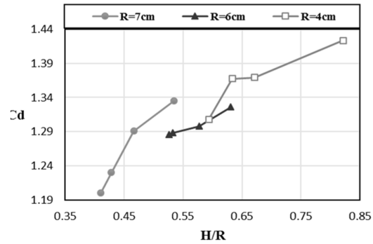
شکل ۱۲- رابطه‌ی بین H/R و C_d .
