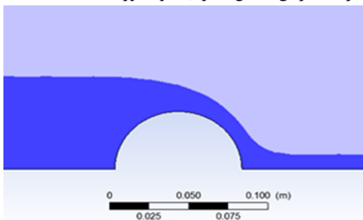
شکل ۶- نیمرخ سطح آب برای شعاع ۴cm و بدهی 0.714 \text{ (l/s)}
