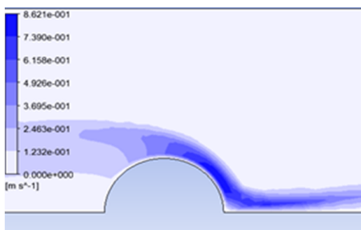
شکل ۷- نمودار توزیع سرعت بر روی سرریز برای شعاع ۴cm و بدهی 0.714 \text{ (l/s)}
