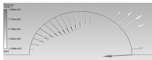
شکل ۱۰- نمودار توزیع فشار بر روی سرریز
