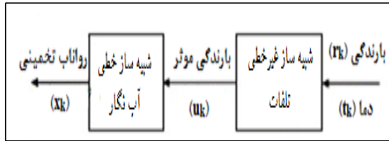
شکل ۲- شبیه‌سازی فرایند بارش- رواناب در شبیه‌ساز IHACRESS
