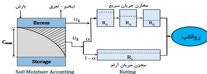
شکل (۴) - نمایش طرح‌واره نرم‌افزار HYMOD.
