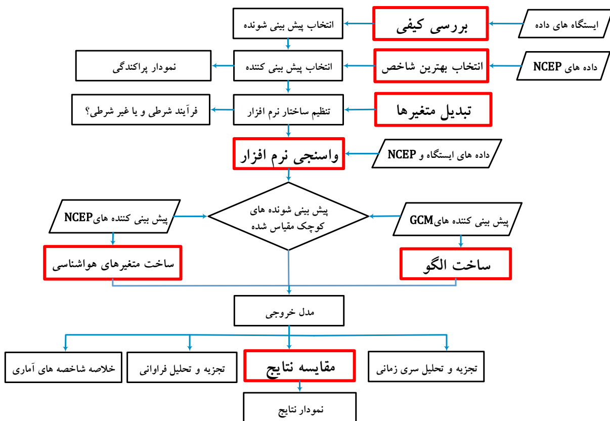
شکل (۲) - نمودار جریان تولید الگوهای اقلیمی بوسیله‌ی نرم‌افزار SDSM (ویلی و همکاران ۲۰۰۷).
