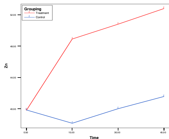
نمودار ۱- میانگین سطح سرمی روی در روزهای صفر، ۱۵، ۳۰، ۴۵ در دو گروه شاهد و تیمار بعد از مصرف مکمل سولفات روی (زمان برحسب روز و روی برحسب میکروگرم بر دسی‌لیتر)
