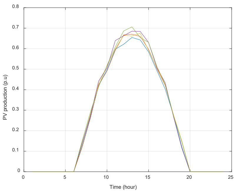
شکل (۳): سناریوهای تولید شده برای منبع PV
