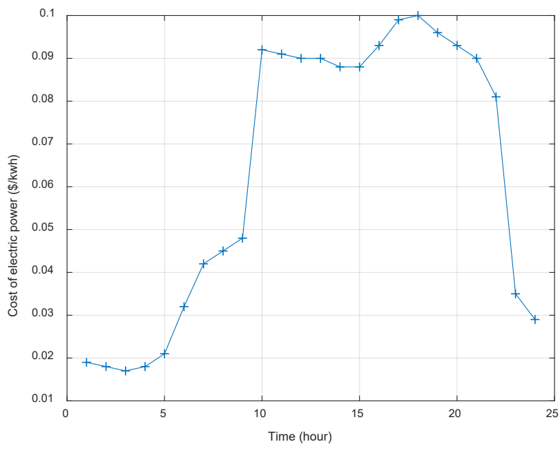
شکل (۴): قیمت انرژی الکتریکی در یک دوره ۲۴ ساعته
