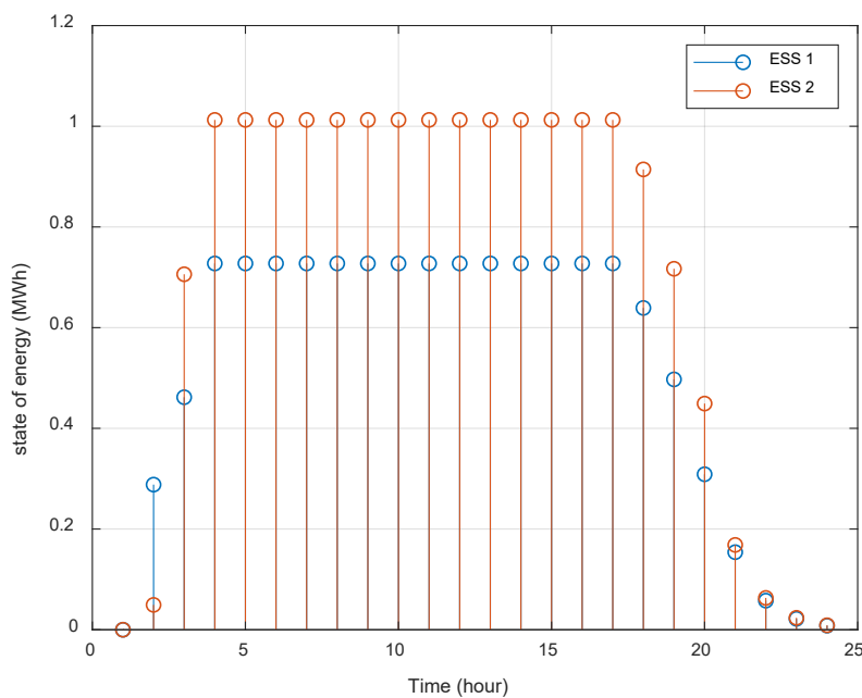
شکل (۹): وضعیت انرژی باتری‌ها در بهره‌برداری جزیره‌ای
