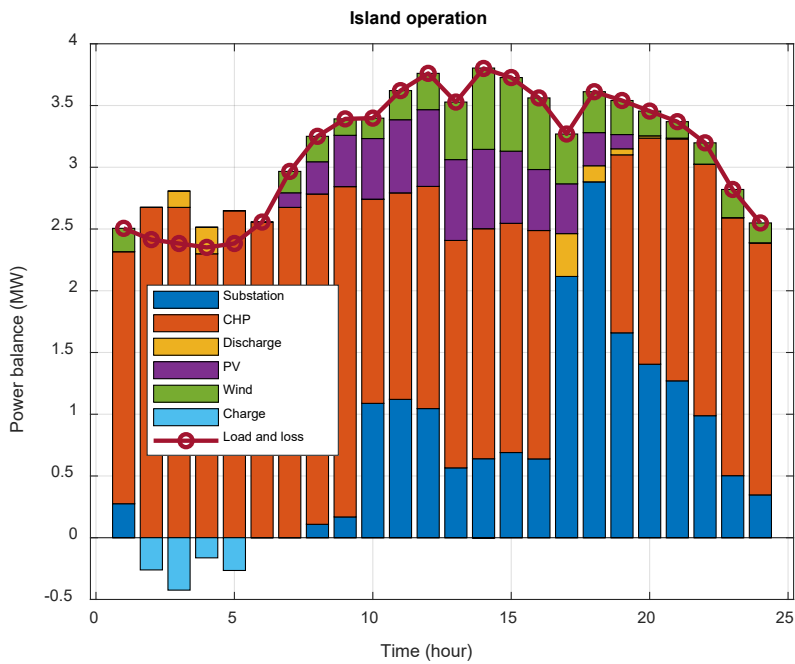
شکل (۱۰): تعادل بار در ریز شبکه ۶۹ باس در حالت بهره برداری متصل به شبکه
