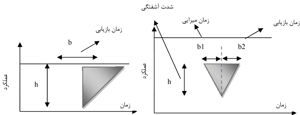
شکل ۱. مثلث تاب‌آوری
