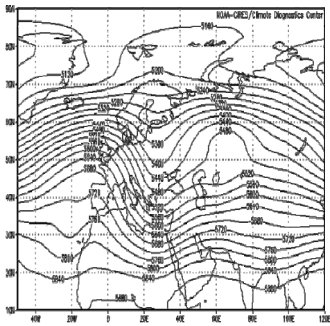
شکل ۴: نقشه سطح ۵۰۰ هکتوپاسکال مارس ۱۹۹۸.
