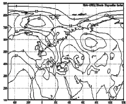
شکل ۵: نقشه انومالی فشار مارس ۱۹۹۸.
