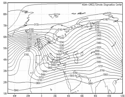
شکل ۱۳: نقشه سطح ۵۰۰ هکتوپاسکال فوریه ۱۹۹۹
