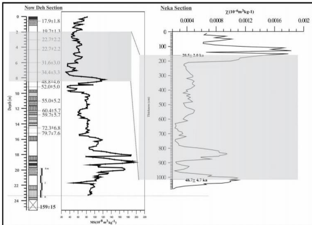
شکل ۴. مقایسه نمودار پذیرفتاری مغناطیسی برش رسوبی نوده و نکا (Feizi et al., 2016).
