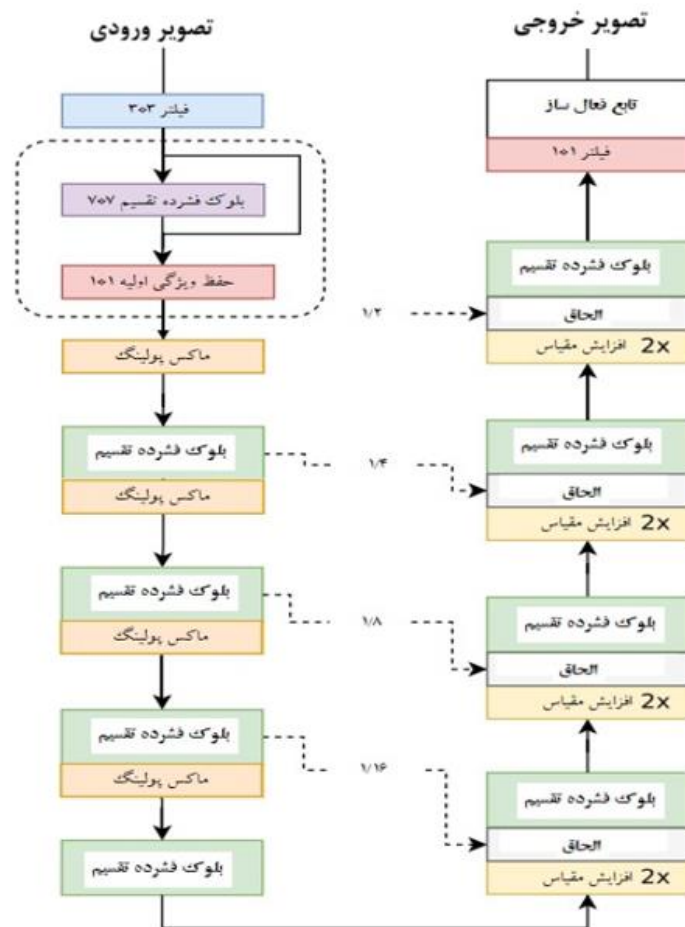
شکل ۳: شبکه قطعه‌بندی عمیق با فشرده‌گی ویژگی‌ها
