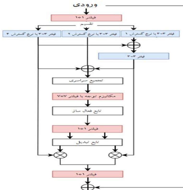
شکل ۲: مازول فشرده سازی توزیع شده Figure 2: Distributed compression module
