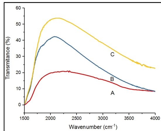
شکل ۴: میزان عبور در بازه عدد موج 400 \text{ تا } 4000 \text{ cm}^{-1} برای نمونه های اسپینل تهیه شده با SPS.
