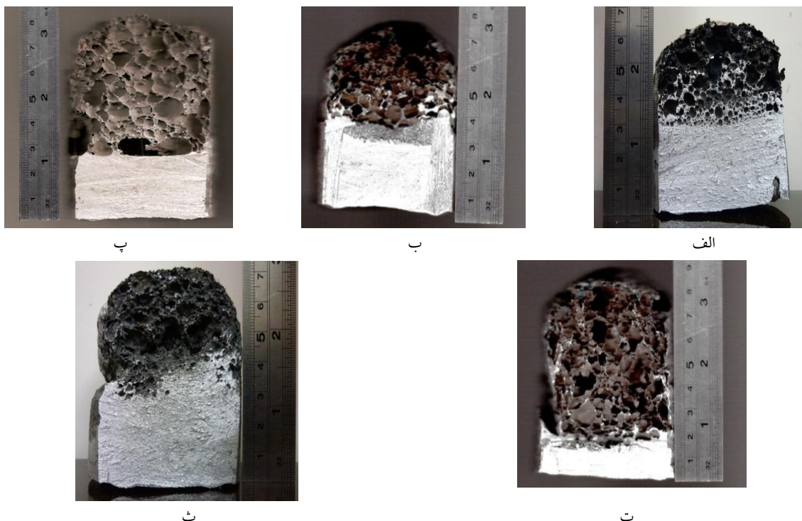
شکل (۶): تصویر مقطع طولی فوم های تولید شده: (الف): آلیاژ آلومینیوم غیر کامپوزیتی، (ب): آلومینیوم + ۰/۲۵٪ وزنی نانوسیلیس، (پ): آلومینیوم + ۰/۵٪ وزنی نانوسیلیس، (ت): آلومینیوم + ۰/۷۵٪ وزنی نانوسیلیس، (ث): آلومینیوم + ۱/۰٪ وزنی نانوسیلیس
