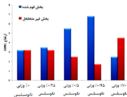
شکل (۷): ارتفاع بخش فوم شده و غیر متخلخل در فوم های تولید شده
