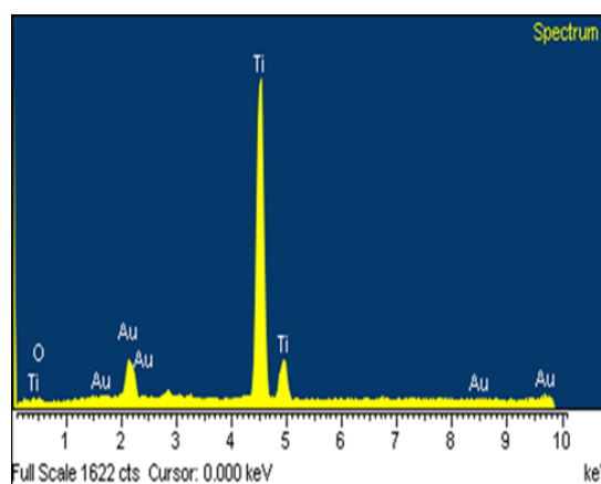
شکل (۳): آنالیز EDS پودرهای هیدرید تیتانیم، بعد از عملیات حرارتی
