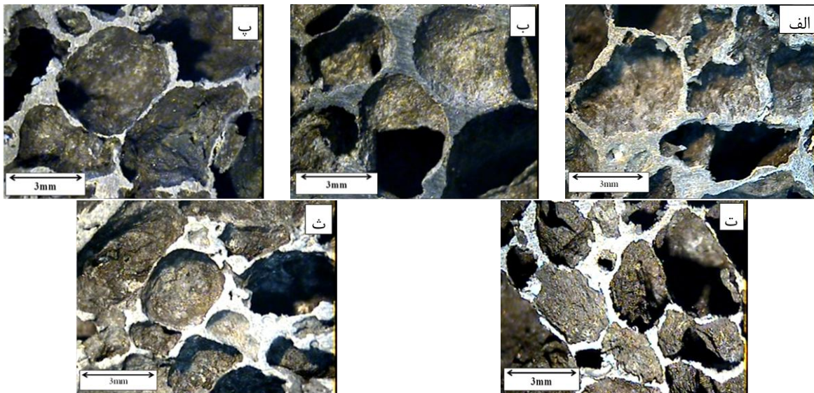
شکل (۱۱): تصویر سطح مقطع عرضی فوم های ساخته شده با ویسکوزیته های مختلف: (الف): آلیاژ آلومینیم غیر کامپوزیتی، (ب): آلومینیم+۰.۲۵٪ وزنی نانوسیلیس، (پ): آلومینیم+۰.۵٪ وزنی نانوسیلیس، (ت): آلومینیم+۰.۷۵٪ وزنی نانوسیلیس، (ث): آلومینیم+۱.۰٪ وزنی نانوسیلیس
