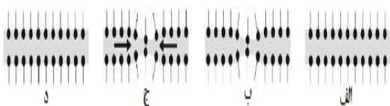
شکل (۸): مکانیزم پایداری دینامیکی فوم ها: (الف): حالت اولیه فیلم نازک، (ب): کشش سطحی موضعی بیشتر، به خاطر نازک شدن موضعی، (ج): گرادیان کشش سطحی، مولکول های سرفکتانت را به سمت قسمت نازک شده می کشد، (د): فیلم اصلاح شده با مکانیزم های انتقال سطح [۲۸]
