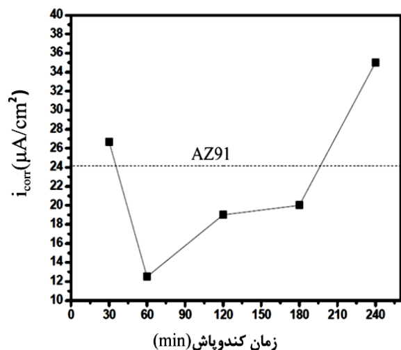
شکل (۱۲): دانسیته جریان خوردگی لایه نیتريدزیر کونیم بر حسب زمان لایه‌نشانی در محلول رینگر
