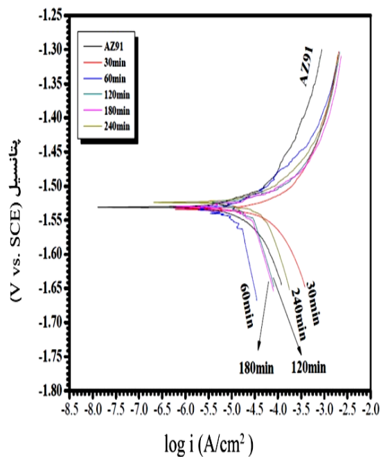
شکل (۱۰): نمودار پلاریزاسیون پتانسیودینامیک آلیاژ AZ91 لایه‌نشانی شده به وسیله نیتريدزیر کونیم در زمان‌های مختلف لایه‌نشانی در محلول رینگر
