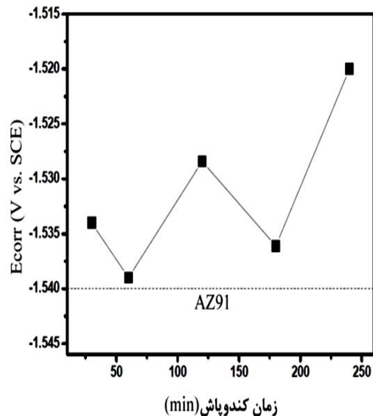
شکل (۱۱): پتانسیل خوردگی لایه نیتريدزیر کونیم بر حسب زمان لایه‌نشانی در محلول رینگر
