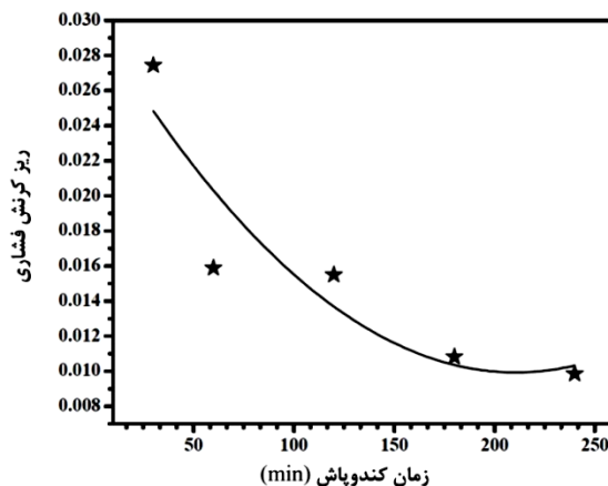
شکل (۷): تغییرات میکروکرنش در لایه نیتريد زیرکونیوم نسبت به زمان لایه نشانی
