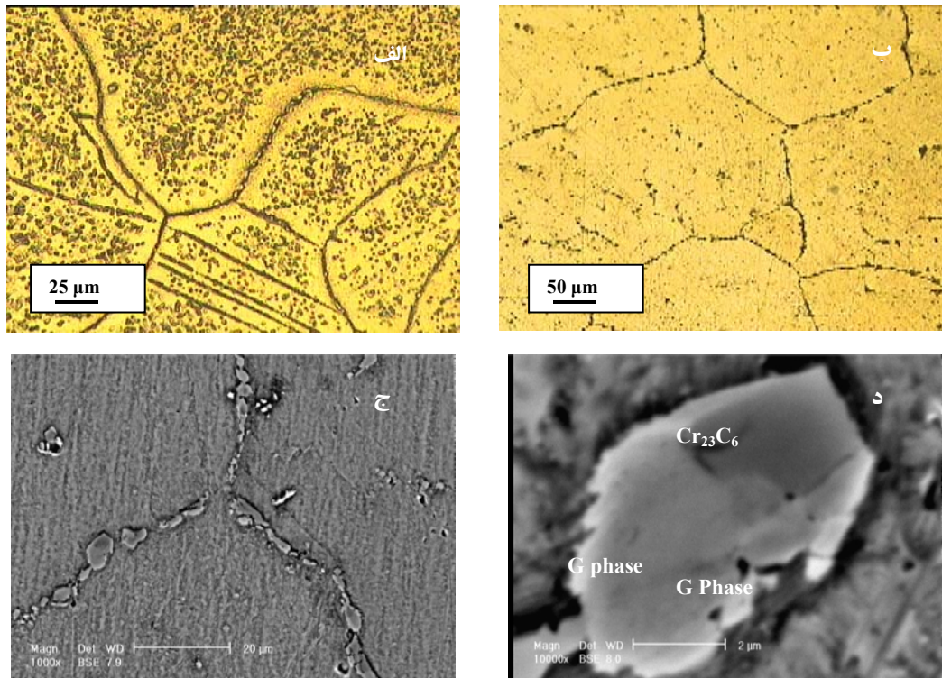
شکل (۲): ریزساختار میکروسکوپی آلیاژ ۸۰۰ (الف): پس از پیر شدن، (ب): بعد از آنیل انحلالی در 1200^{\circ}\text{C} ، (ج): تصویر میکروسکوپ الکترونی از رسوبات آلیاژ ۸۰۰ و (د): تصویر میکروسکوپ الکترونی از رسوبات دو رنگی.
