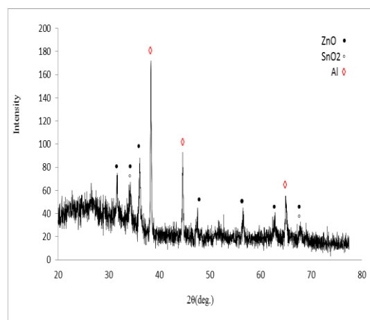
شکل (۲): پراش پرتو X نانو الیاف هسته-پوسته SnO 2 - ZnO
