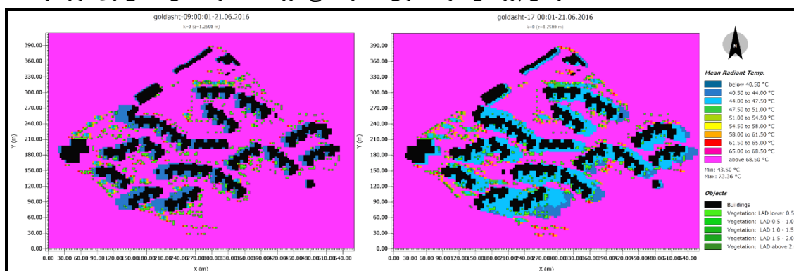
شکل ۷- توزیع دمای متوسط تابشی، ۹ صبح (چپ) و ۱۷ بعدازظهر (راست). منبع: یافته‌های تحقیق، ۱۳۹۵.
