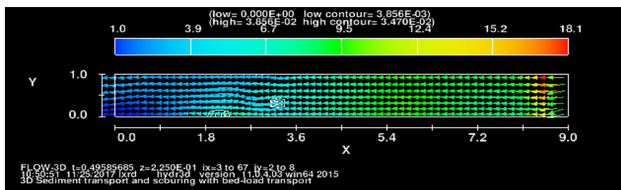
شکل ۵- تغییرات دبی در جریان مدل سازی شده فلوم در مدل پل با طوقه ال شکل
