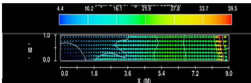
شکل ۶- تغییرات دبی در جریان مدل سازی شده فلوم در مدل پل بدون طوقه ال شکل
