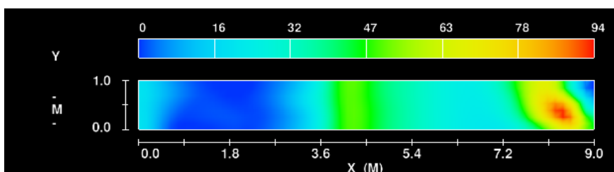
شکل ۸- تغییرات لزجت سیال در مدل سازی شده فلوم در مدل پل بدون طوقه ال شکل
