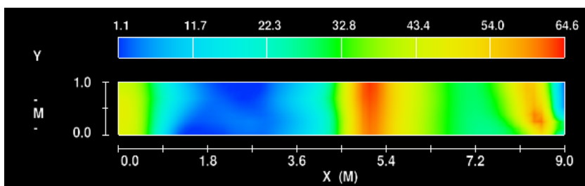
شکل ۷- تغییرات لزجت سیال در مدل سازی شده فلوم در مدل پل با طوقه ال شکل ۳
