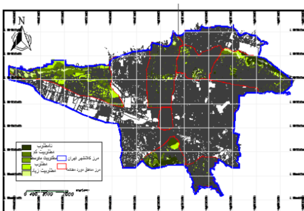
شکل ۳ - نقشه مطلوبیت مناطق مورد مطالعه حاصل از مدل باینری مأخذ: یافته های نگارنده، ۱۴۰۳
