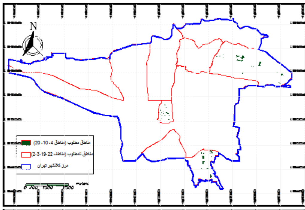
شکل ۲ - نقشه مطلوبیت مناطق مورد مطالعه حاصل از منطق بولین مأخذ: یافته های نگارنده، ۱۴۰۳
