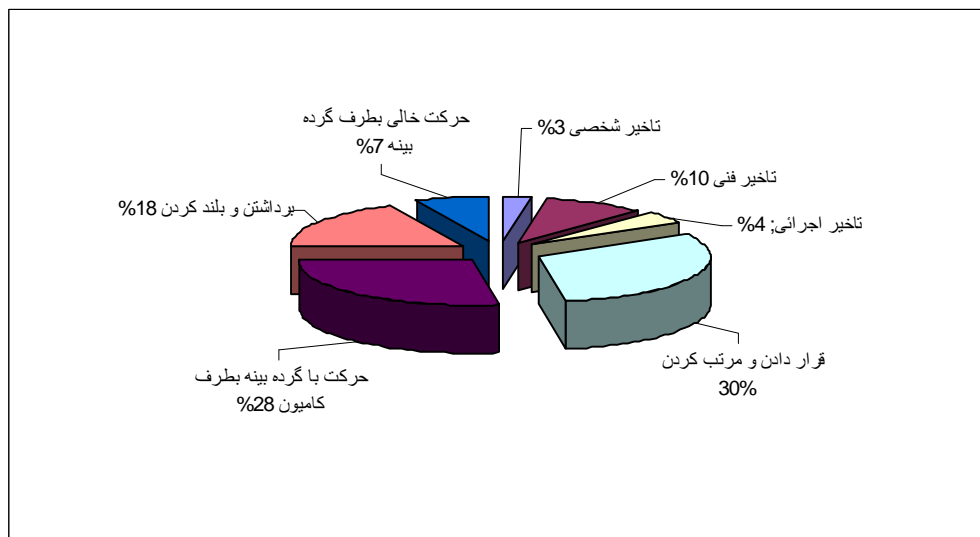
شکل ۱- درصد زمان صرف‌شده به‌وسیله اجزای یک نوبت بارگیری بالودرچنگک‌دار با احتساب زمان تاخیر
