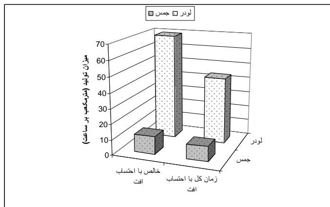
شکل 3- میزان تولید (مترمکعب بر ساعت) دو دستگاه بارگیری لودر چنگک دار و جمس با احتساب تاخیر و بدون آن
