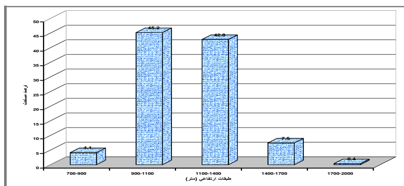
شکل ۱۰. وضعیت طبقات ارتفاعی اراضی در دهستان وکیل آباد
