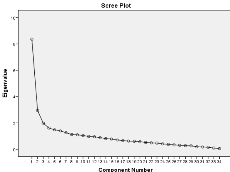
نمودار ۱. نمودار شیب دامنه عوامل (اسکری پلات)
