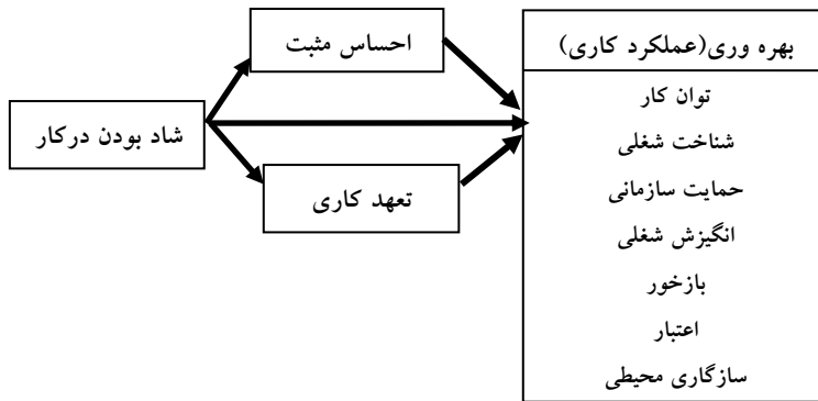
شکل ۱. مدل تحقیق
