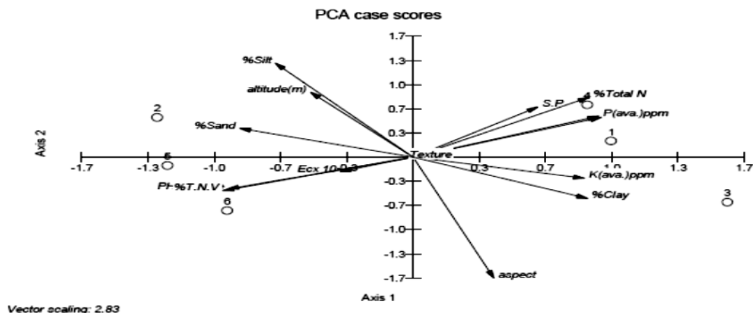
شکل ۱- ارتباط فاکتورهای محیطی و پلات های مختلف بر اساس محور ۱ و ۲ در گونه بارانک
