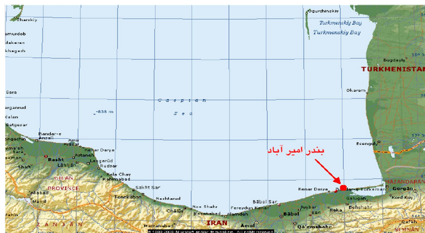
شکل ۱- موقعیت جغرافیایی بندر امیرآباد در خزر جنوبی
