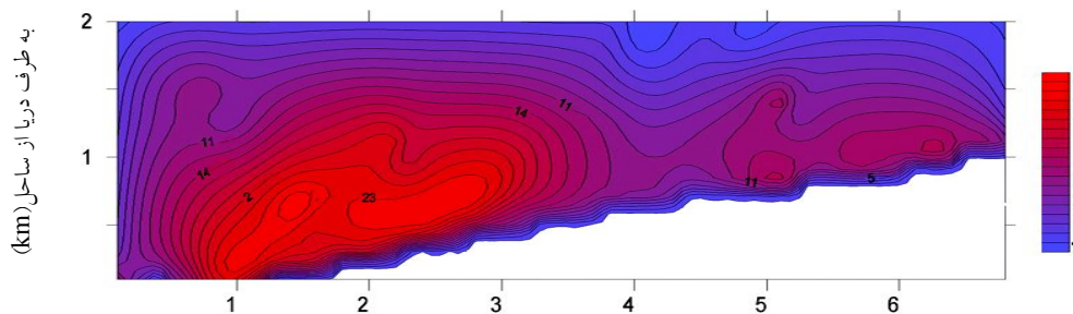
شکل ۳- توزیع تابع جریان (با بزرگنمایی 10^4 ) در منطقه امیرآباد در ماه هشتم (۱۳۸۶) و لایه اول (واحد تابع جریان \frac{m^2}{s} )
