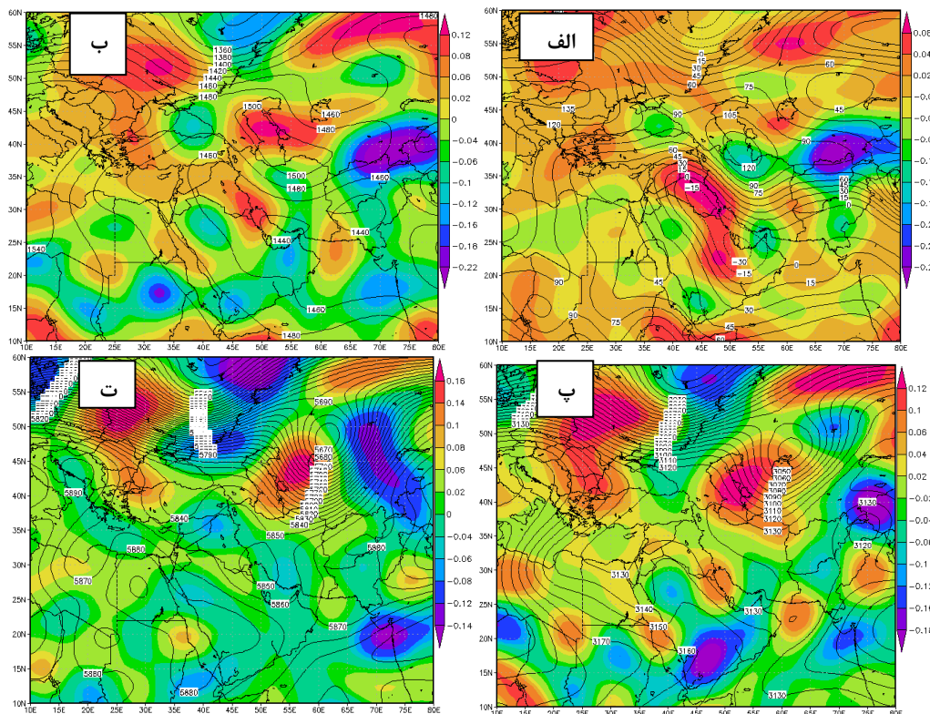
شکل ۱۰: نقشه‌های امگا برحسب پاسکال بر ثانیه در ترازهای الف: ۱۰۰۰، ب: ۸۵۰، پ: ۷۰۰ هکتوپاسکال، ت: ۵۰۰ هکتوپاسکال در روز ۳۰ تیر ۹۴ (منبع نگارندگان)
