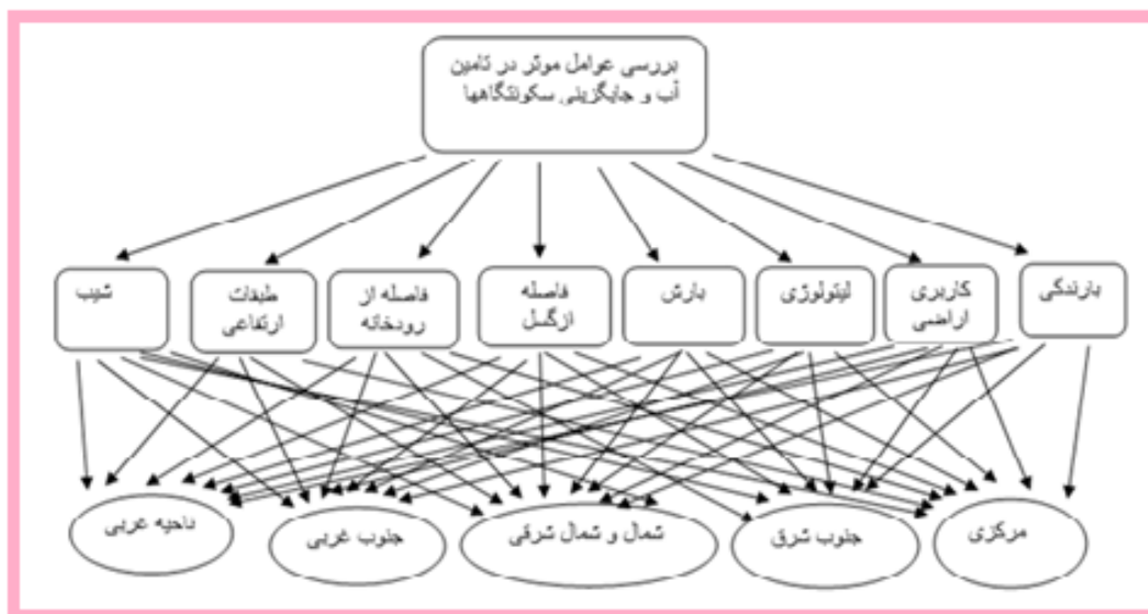
شکل ۱۳: ساخت سلسله‌مراتبی الویت بندی عوامل مؤثر در تأمین آب دشت میاندوآب
