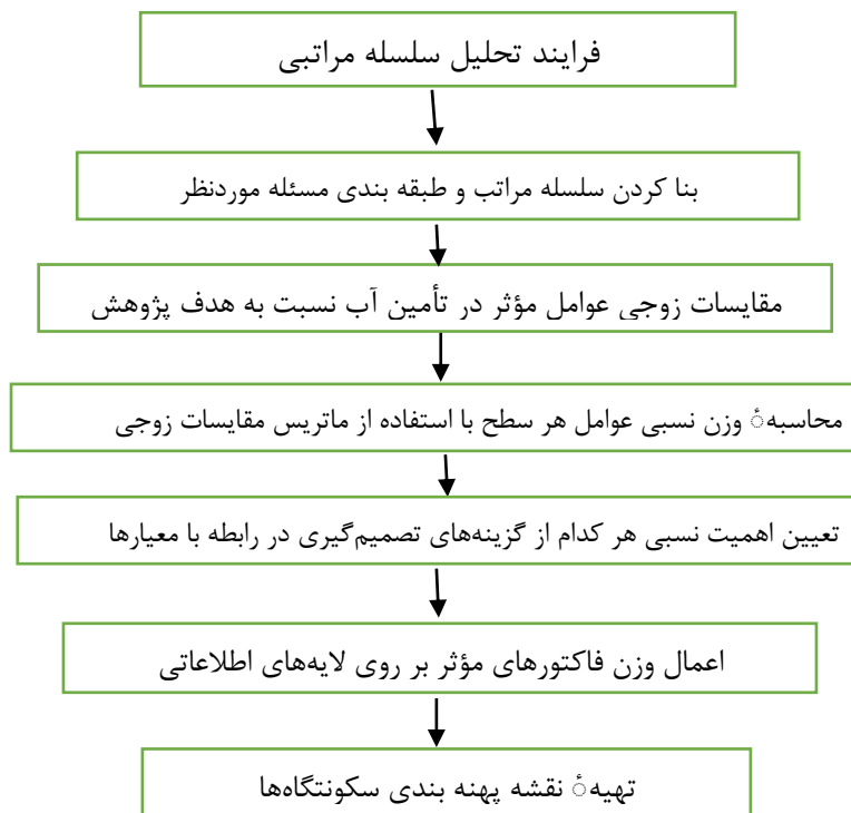
شکل ۱: فلوچارت مراحل فرایند تحلیل سلسله‌مراتبی
