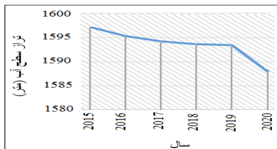
شکل ۸. هیدرو گراف تغییرات زمانی تراز آب چاه‌های مشاهداتی سال ۲۰۱۵ تا ۲۰۲۰
