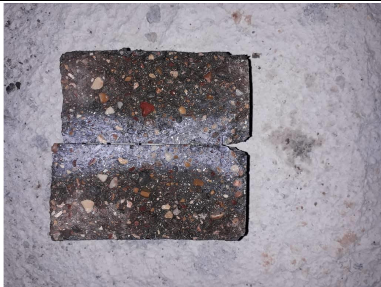
شکل ۴. پاشش نیترات نقره و تغییر رنگ ناحیه نفوذ کرده
