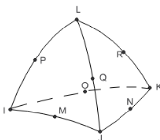
شکل ۸. نمای شماتیک المان مورد استفاده
