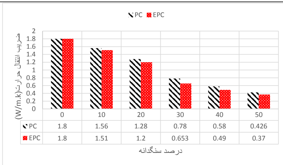
شکل ۱۷. ضریب انتقال حرارت مخلوط‌ها (وات بر متر کلوین)
