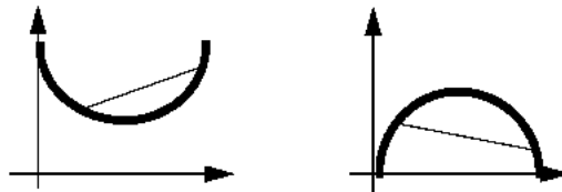
شکل ۲ - کمینه‌سازی با تابع هدف درجه دوم محدب و بیشینه‌سازی با تابع هدف درجه دوم مقعر
