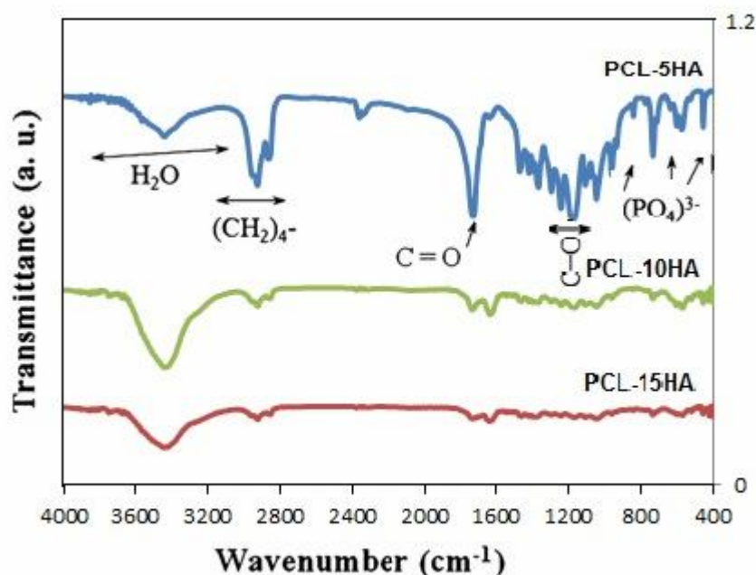
شکل ۲- الگوی آزمون طیف‌سنجی فرسرخ با تبدیل فوریه داربست‌های کامپوزیتی پلی کاپرولاکتون- هیدروکسی آپاتیت تهیه شده با درصد وزنی گوناگون از هیدروکسی آپاتیت
