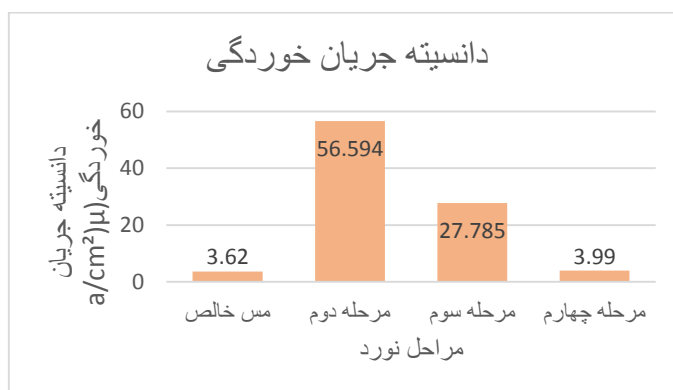
شکل ۱۴- نمودار دانشیته جریان خوردگی مس/اکسید گرافن در پاس‌های مختلف نورد و مس خالص ARB شده در پاس‌های مختلف
