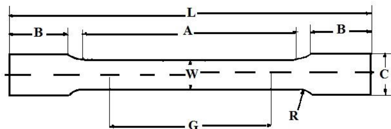
شکل ۲- شماتیک نمونه ای آزمون کشش بر اساس استاندارد ASTM E8M
