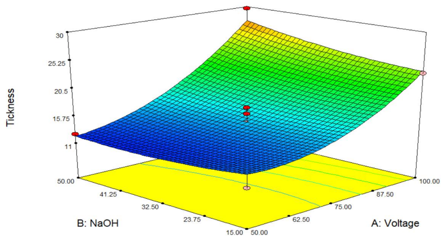
شکل ۳- نمودار سه بعدی تغییرات NaOH و ولتاژ بر حسب سختی در زمان ثابت
